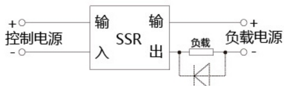
接线图
