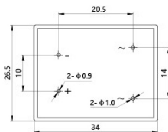
安装尺寸
